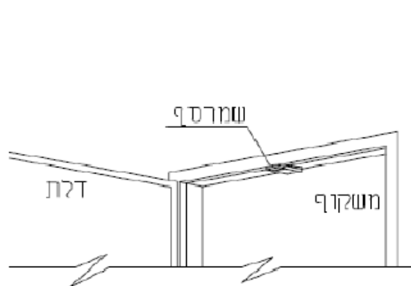
פרט 9 חלק עליון של הדלת
